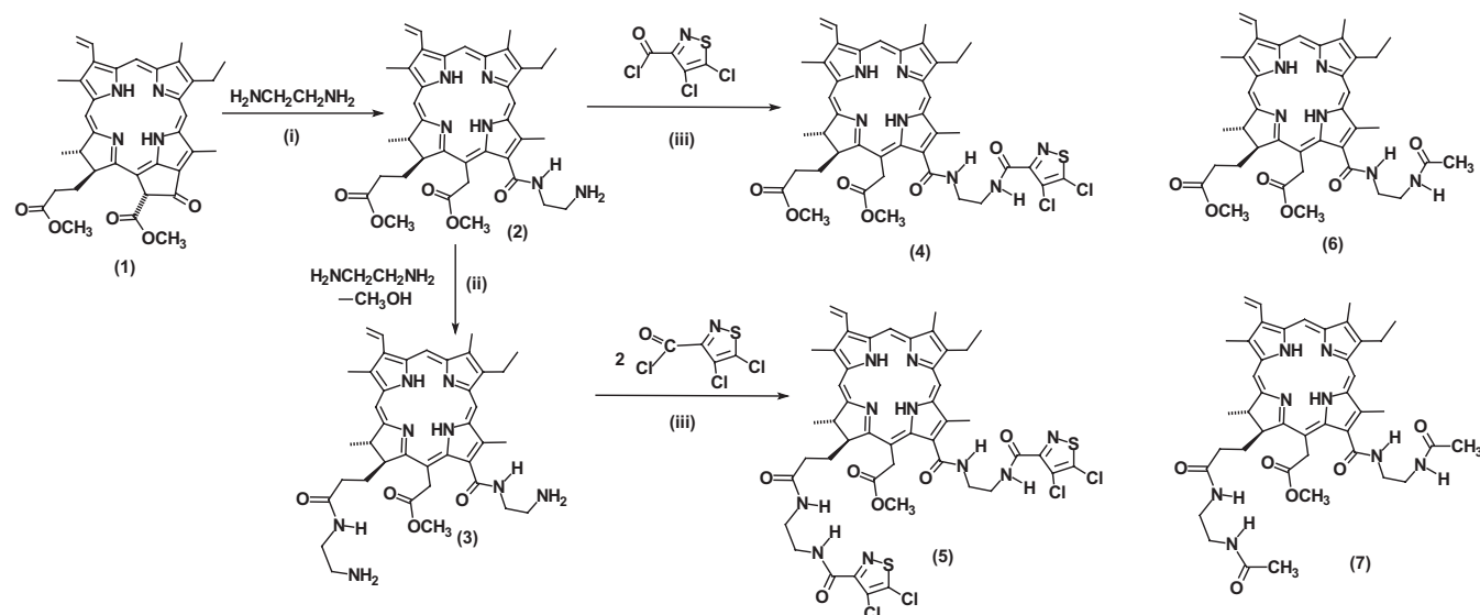
Схема 1. Синтез производных хлорина e_6 с одним и двумя фрагментами хлоризотиазола.
