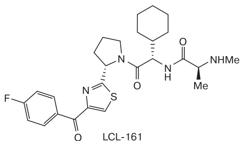
LCL-161
