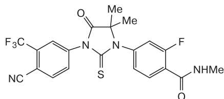
Enzalutamide
