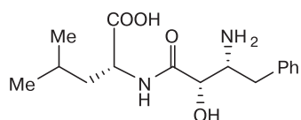
Bestatin
